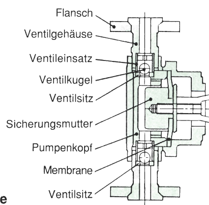
Modell BZ1X, 3X, 5X
