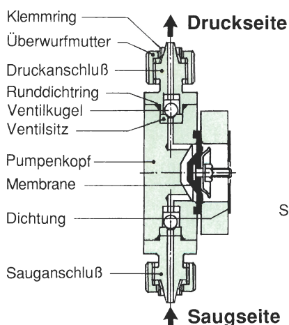
Modell BA01 - 50
