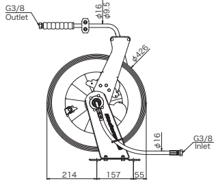
801428 LBM-G, 801237 LBM-16 802238 LBM-30, 801429 LBM-60
