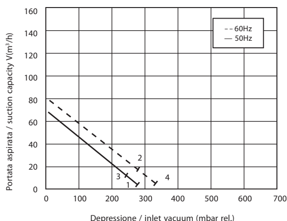
ASPIRAZIONE / EXHAUST
