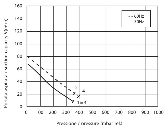
COMPRESSIONE / COMPRESSION
