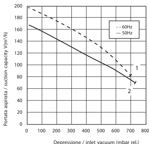
ASPIRAZIONE / EXHAUST
